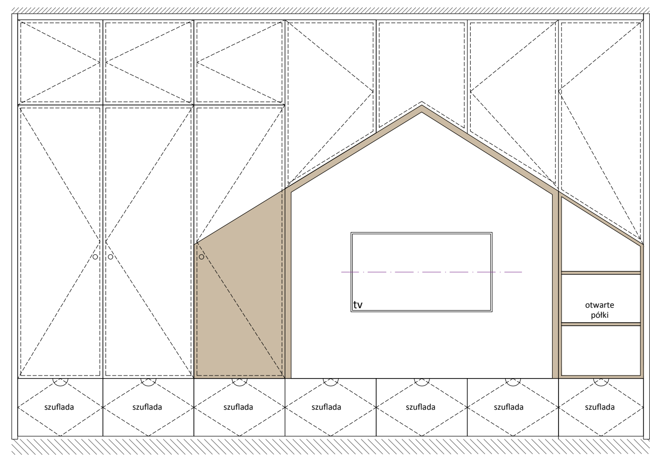
Funkcjonalność mebla została przygotowana zgodnie z rysunkiem poglądowym. Dolna część składa się z rzędu wysokich szuflad, górna to drążki i półki z możliwością regulacji wysokości
